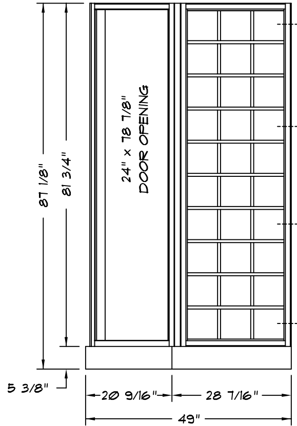
ELEVATION B
