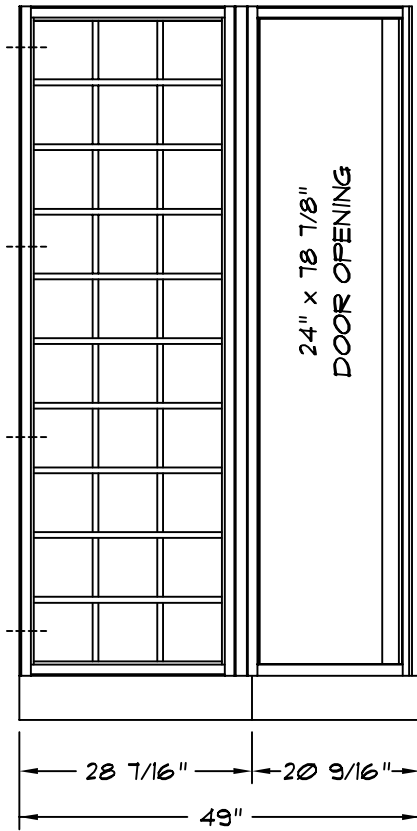
ELEVATION A
