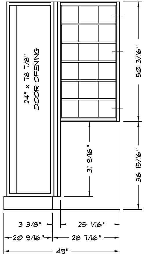
ELEVATION B
