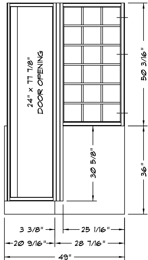
ELEVATION B
