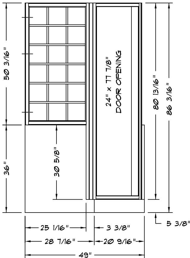
ELEVATION A
