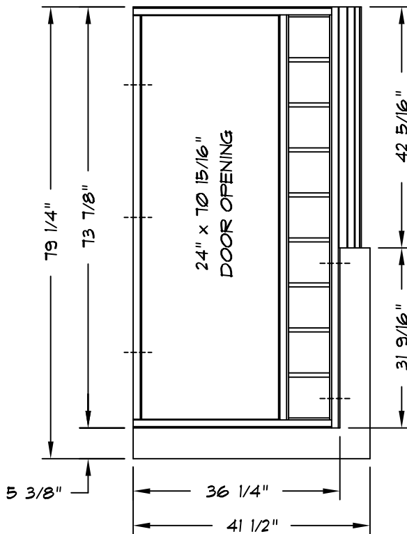
ELEVATION A
