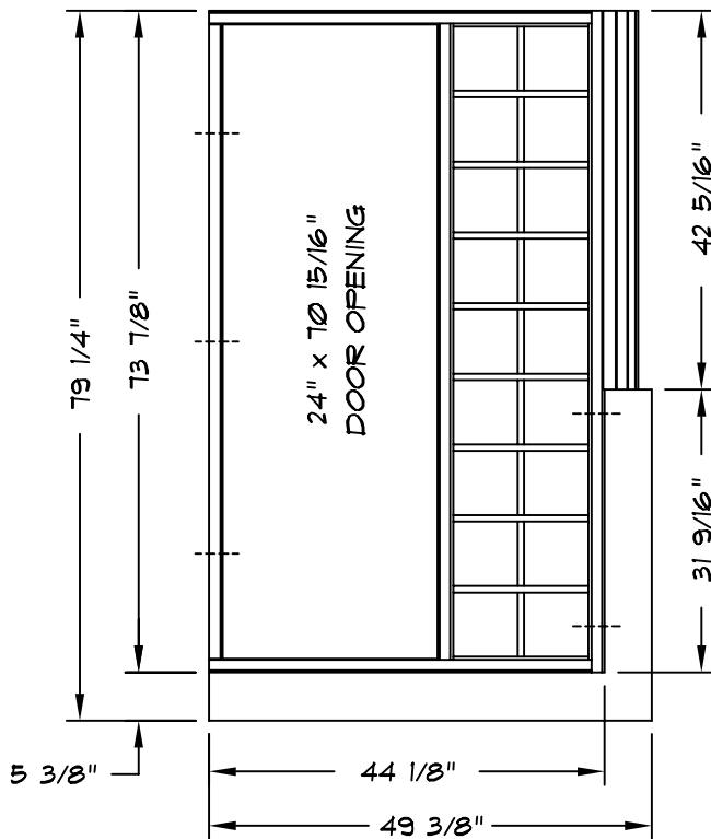
ELEVATION A
