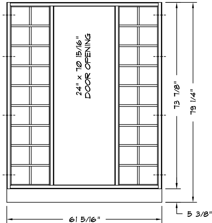
ELEVATION
